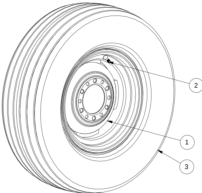
9.5L-15 TIRE & RIM (55-082-026)
