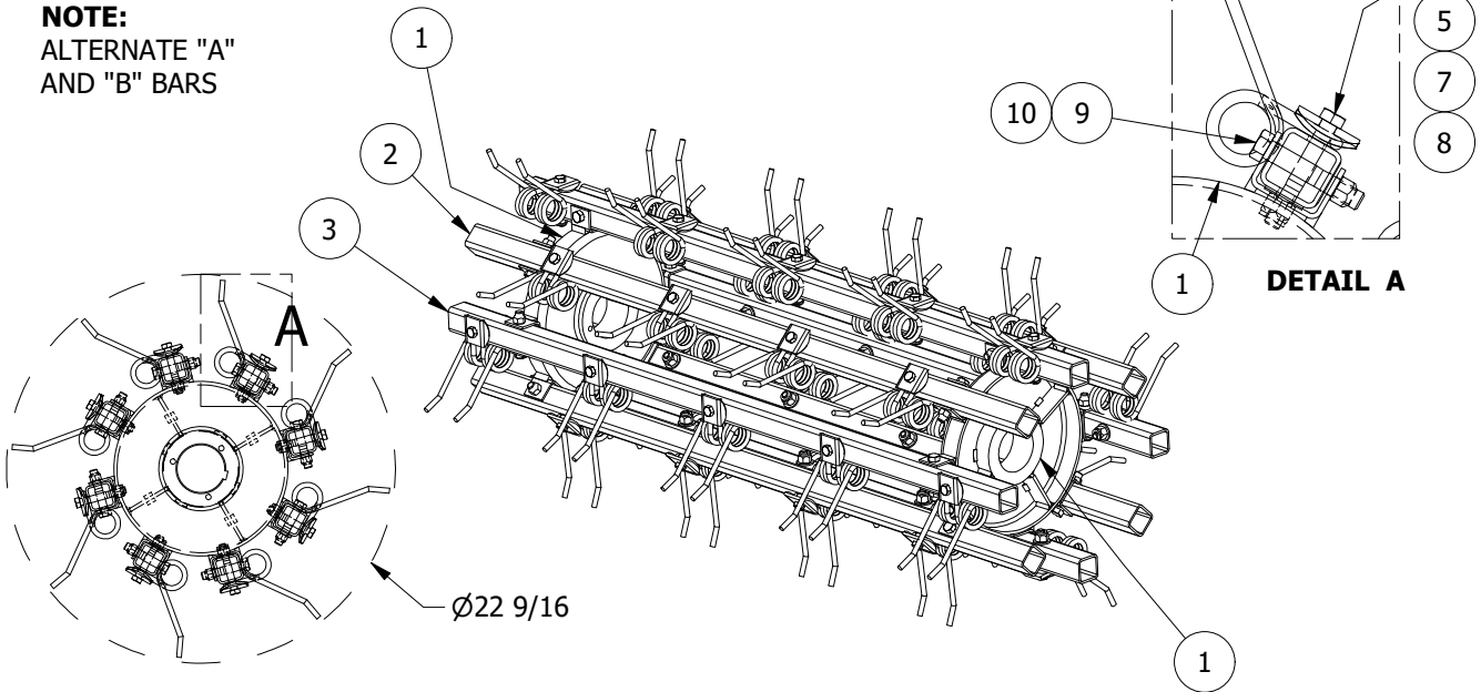
SECTION A-A
